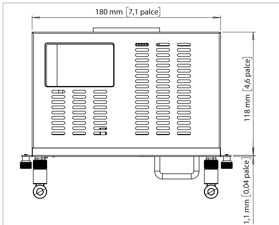
Pohled shora
