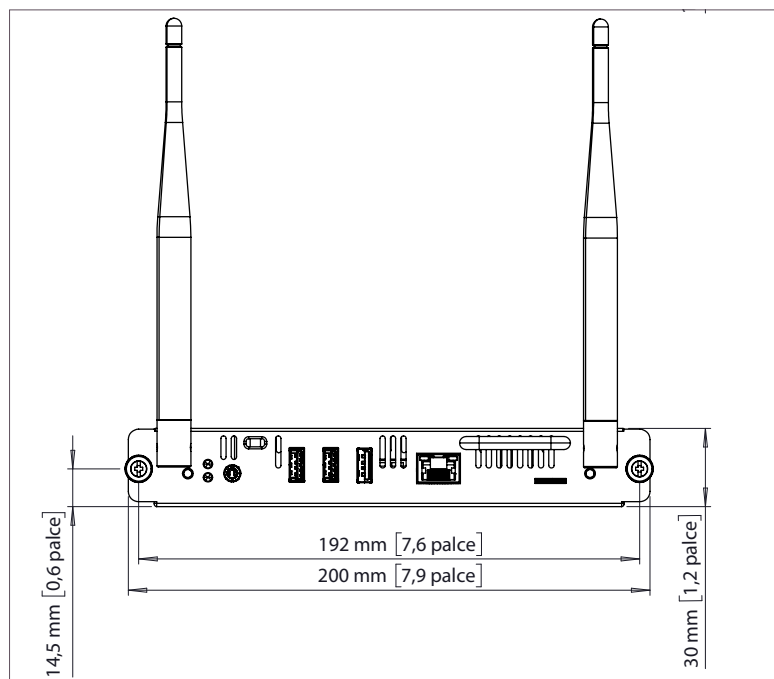
Pohled zepředu
