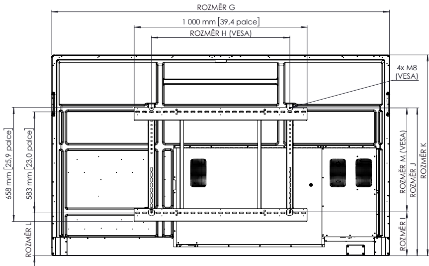
Pohled zezadu
