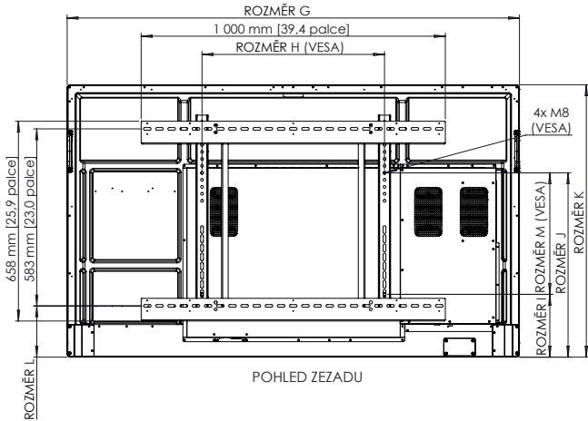
Pohled zezadu
