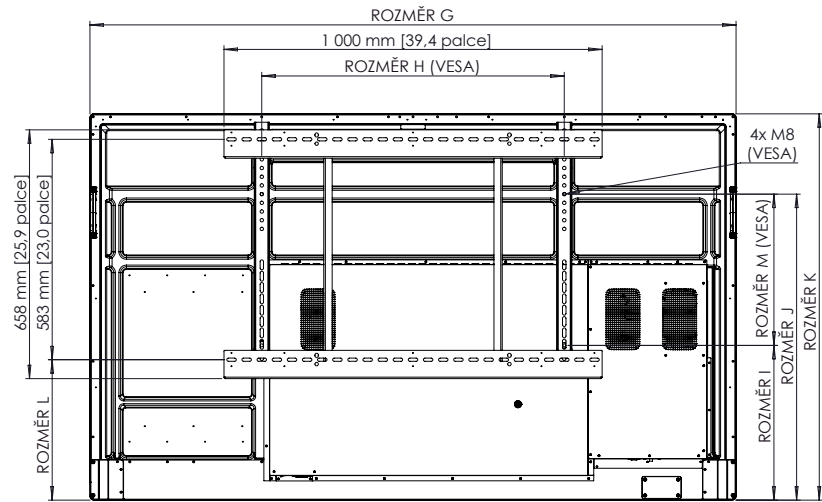
Pohled zezadu
